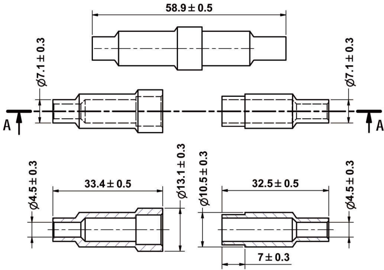
A-A 剖視圖:
